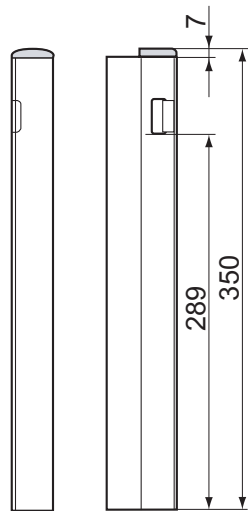
Edge cap, 350 mm, right
