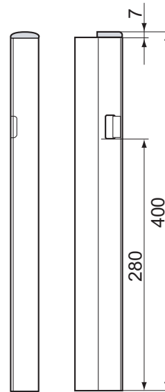
Edge cap, 400 mm, right
