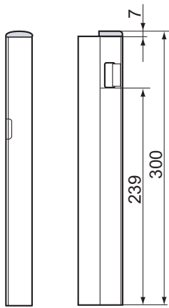
Edge cap, 300 mm, right
